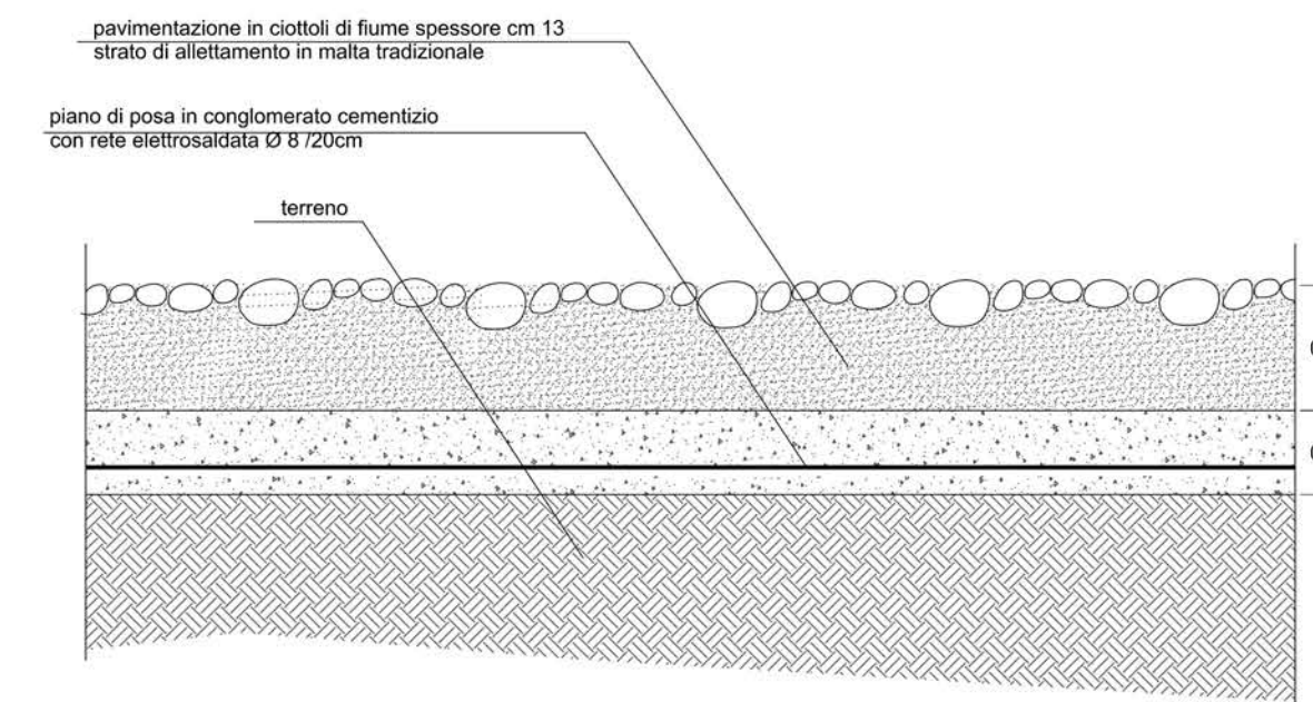
Particolare pavimentazione in acciottolato scala 1:10
